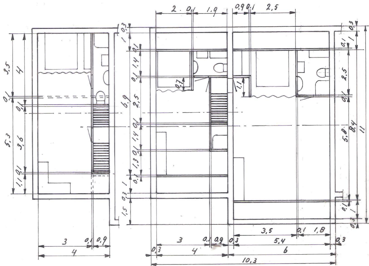
figuur 2 Bovenaanzicht 1° studio (links) en bovenaanzicht 2° studio en 3° studio op de zolders (rechts)
