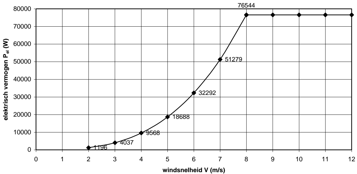
Figuur 1 Geschatte P_{el} - V kromme voor een windturbine met een rotordiameter D = 30 m
