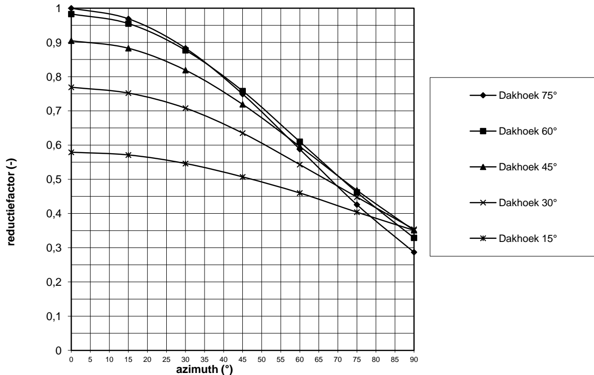
Figuur 1 Reductiefactor als functie van de dakhoek en de azimuth t.o.v. een paneel met een dakhoek van 75° en een azimuth van 0° voor de maand december
