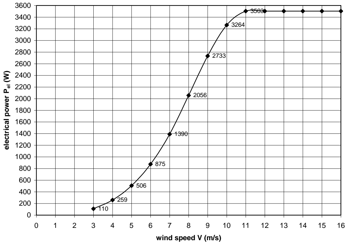
fig. 1 P_{el} - V kromme VIRYA-5B3 voor een inverter belasting
